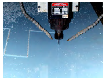
Fresadora automàtica 3000/1540
