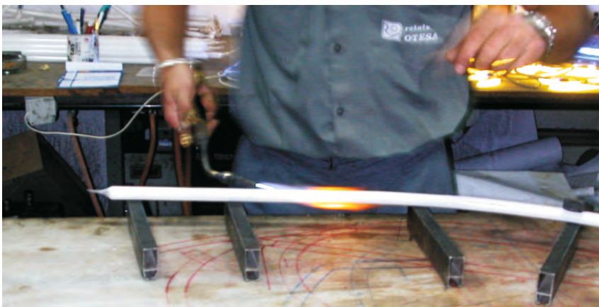
Curvat del neó amb bufador
